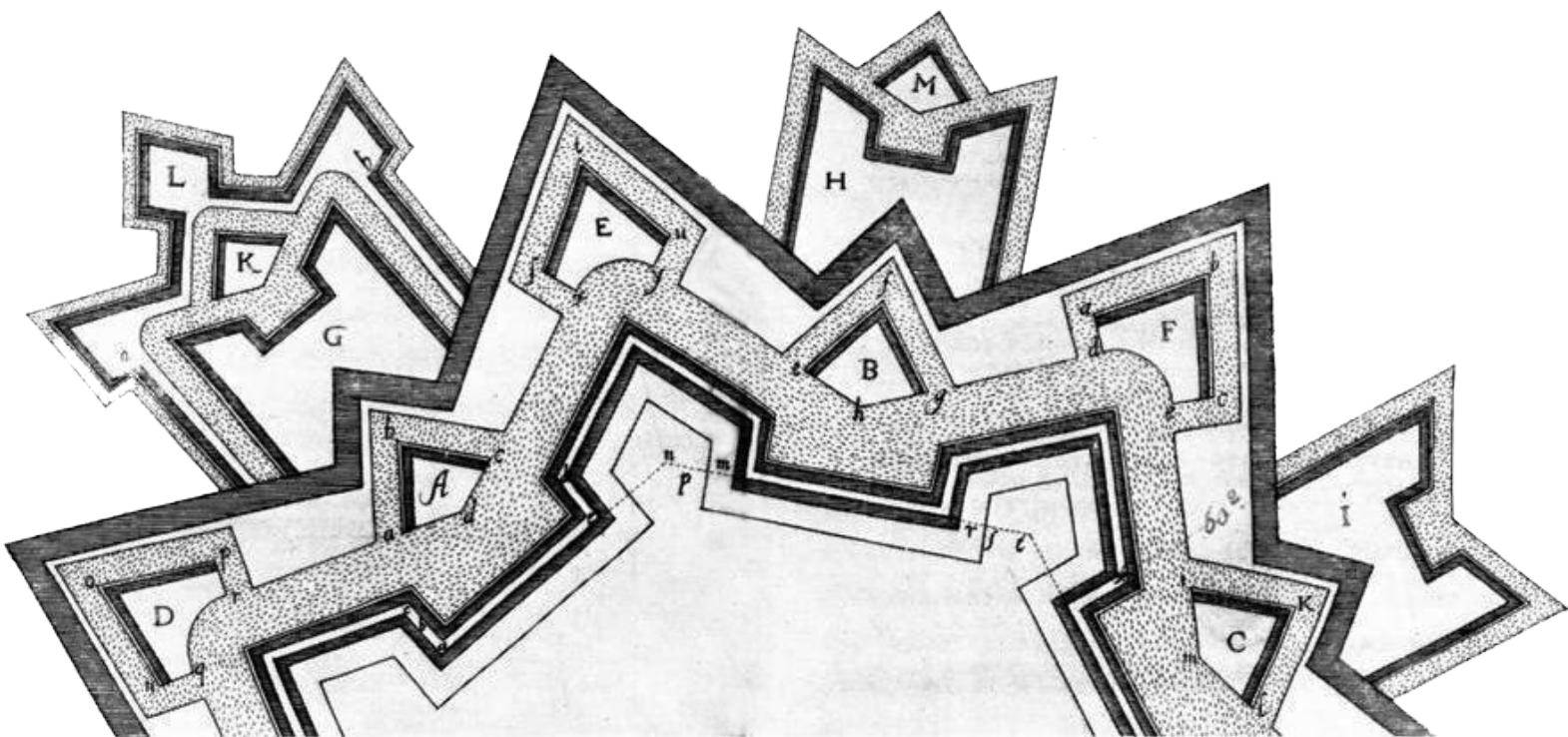
Plano de una sección del sistema defensivo abaluartado. Dibujo proveniente del libro Architectura militaris , del ingeniero Adam Freitag, publicado en 1631. Podemos ver la estructura de las siguientes obras defensivas: Revellines: A, B, C, K, L y M. Media-lunas: D, E y F. Hornabeques: G, H y I. El sistema se basa en una eficaz combinación de defensa avanzada y solapamiento de protección por el fuego: la fortaleza –con sus tres bastiones– proporciona cobertura de fuego a las obras exteriores, que se van expandiendo hacia el exterior en sucesivas líneas defensivas radiales, protegidas por fosos, escarpas y caminos cubiertos.
