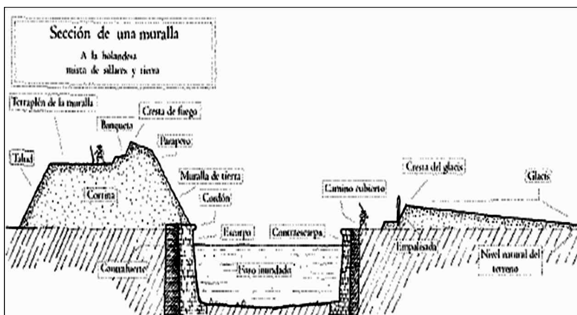
Sección transversal de una muralla abaluartada
