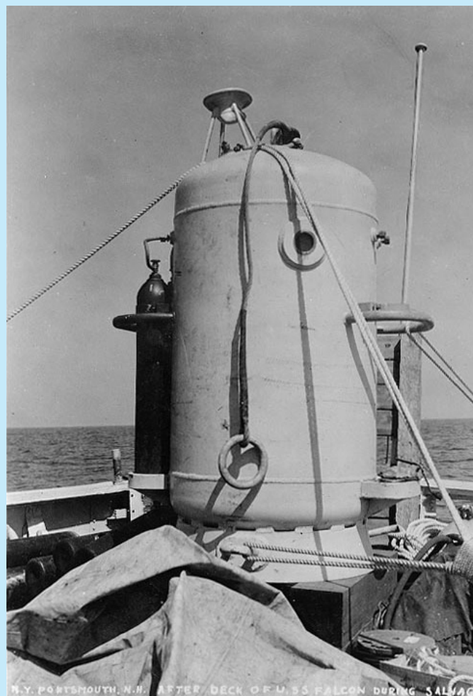
Campana de rescate usada en el incidente del Squalus
