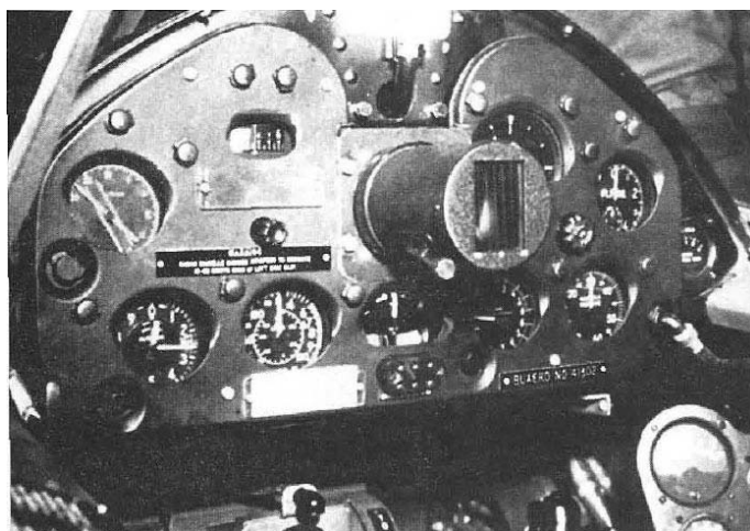
Panel de Control de un caza nocturno F6F-3N Hellcat. Nótese la pantalla de radar de forma cilíndrica en el centro del panel de mandos.
